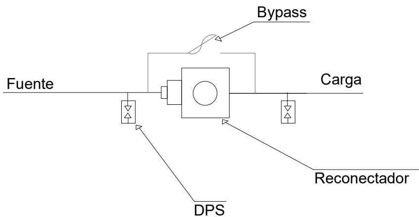
Diagrama unifilar- instalación reconector
